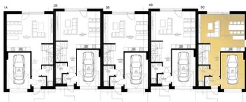
RZUT PARTERU
