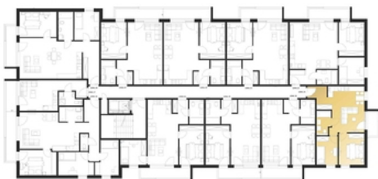
RZUT 2 PIĘTRA
