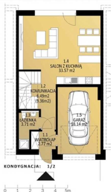
RZUTY BUDYNKU BUDYNEK: 3B
