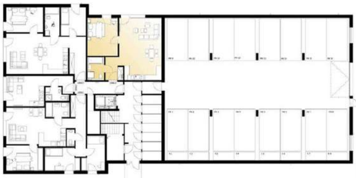
RZUT PARTERU
